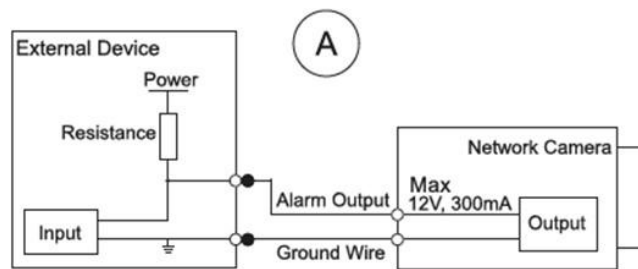
Afbeelding 1-3 Modus A
