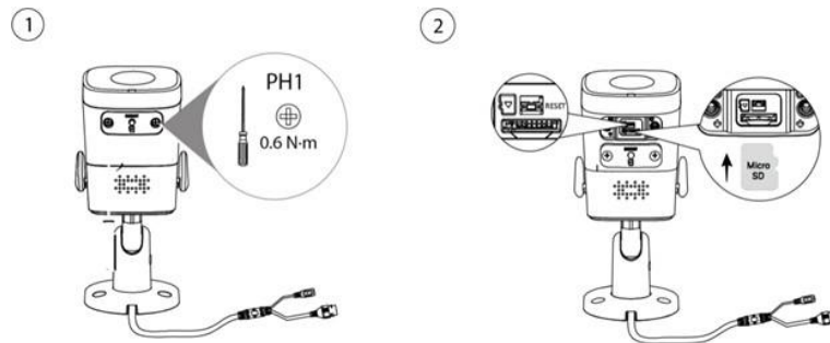
Afbeelding 3-2 Een SD-kaart installeren (eenheid: mm[inch])
