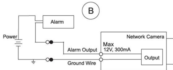
Afbeelding 1-4 Modus B
