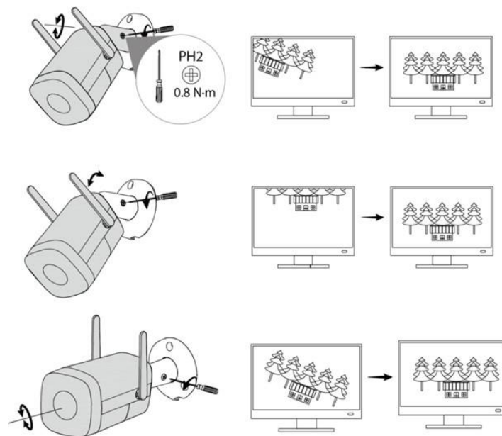
Figuur 3.5 De lenshoek aanpassen
