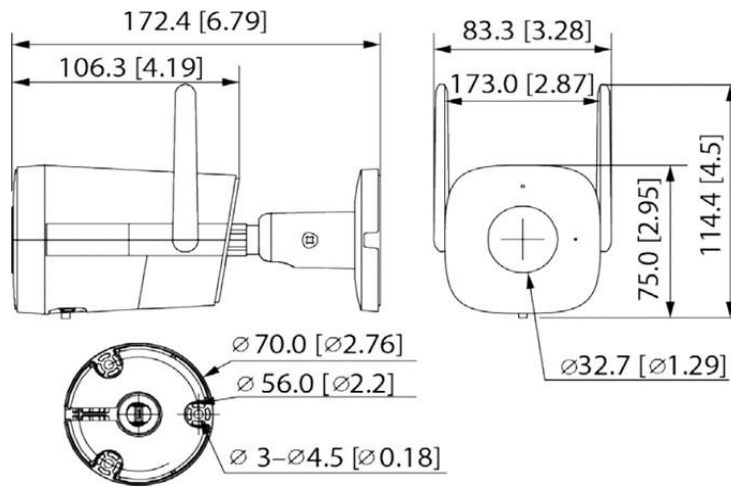
Figuur 3-1 Afmetingen (Eenheid: mm [inch])
